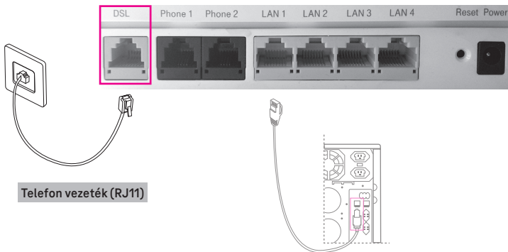
Telefon fali csatlakozó
