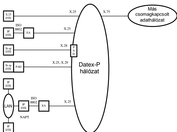
A Datex-P hálózat jellemző elérési módjai
